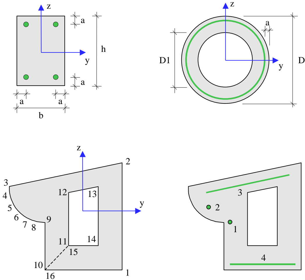
Рис. 1. Сечения
