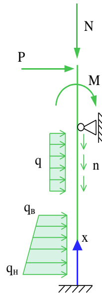
Рис. 2. Положительные направления нагрузок
