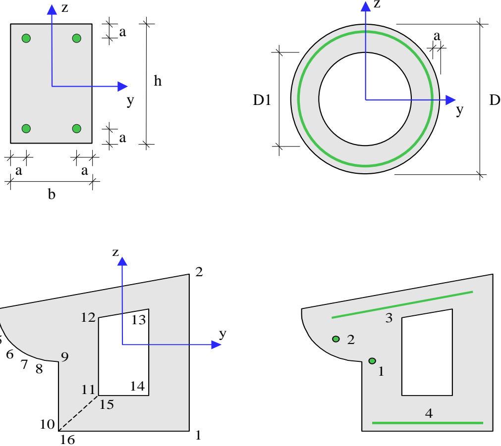
Рис. 4. Сечения
