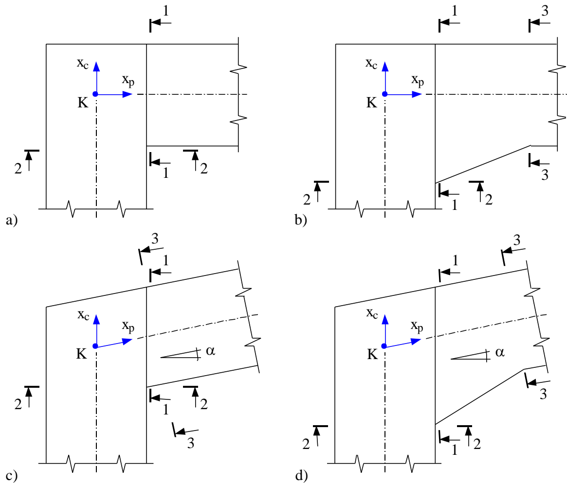
Рис. 4. Сечения узла
