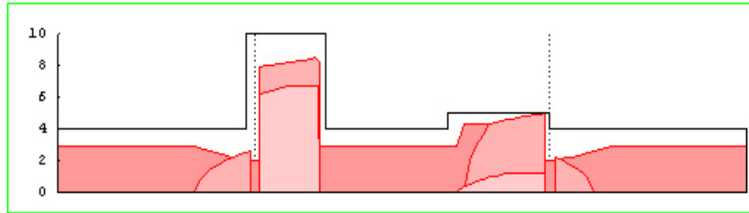
схема армирования сечения с координатой x = 7.23
