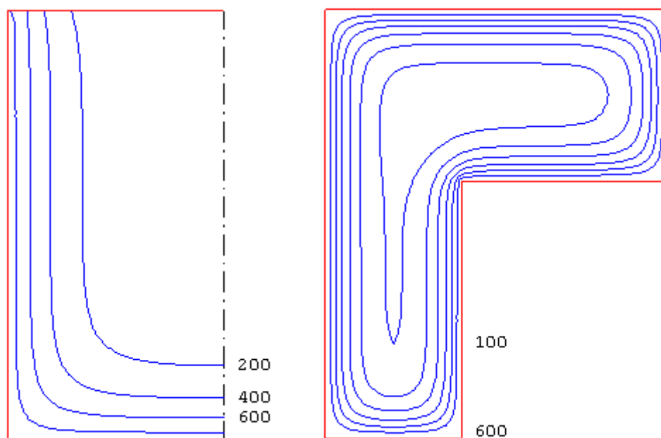
Рис.6. Изотермы
