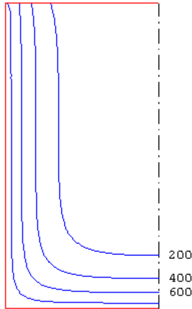
Рис.8. Изотермы
