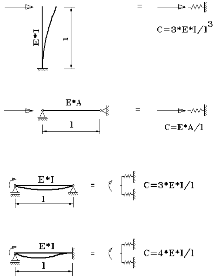
Рис. 2. Коэффициенты жесткости упругих связей
